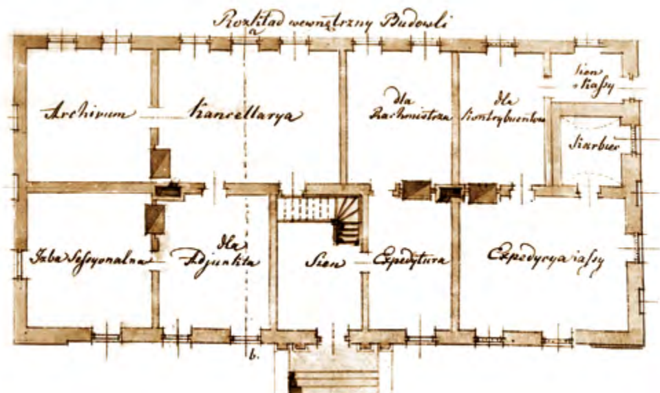
Projekt budynku władz powiatowych i obwodowych z 1837 r. (niezrealizowany). Projekt Domu murowanego na Biuro i Kasę Obwodu Stanisławowskiego pobudować się mający w Mieście Mińsku. Elewacja od frontu. Rozkład wewnętrzny Budowli.
